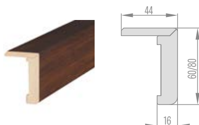
STANDARDNÍ ÚHELNÍK K REGULOVANÉ ZÁRUBNĚ
