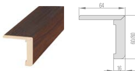
ÚHELNÍK S PRODLOUŽENÝM PEREM K REGULOVANÉ ZÁRUBNĚ
