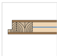
KŘÍDLO 46 mm vyztužené ocelovým plechem
